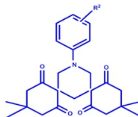
Spiropiperidines
